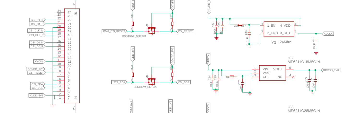
CSI_Interface
